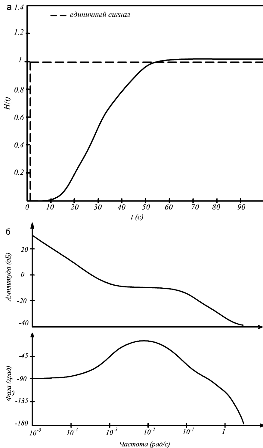
Рис. 2. Переходная (а) и логарифмически-частотные (б) характеристики замкнутой САУ монотонного типа
