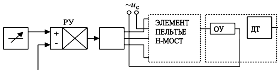
Рис. 1. Функциональная схема САУ терморегулятора (ПУ – регулирующее устройство, ОУ – объект управления, ДТ – датчик температуры)
