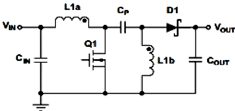
Рис. 1. Преобразователь SEPIC
