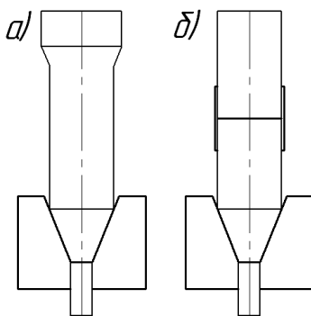
Рис. 6. а) утолщенная в конце заготовка, б) непрерывное прессование
