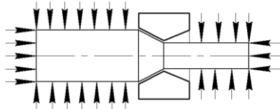
Рис. 4. Гидропрессование с противодавлением
