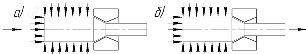
Рис. 3. а) усиленное гидропрессование, б) гидропрессование с волочением
