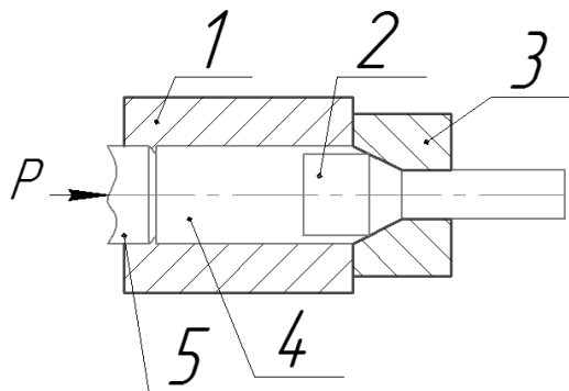
Рис. 1. Схема профиля гидропрессования, где 1 — контейнер, 2 — заготовка, 3 — матрица, 4 — жидкая среда, 5 — пресс-штемпель
