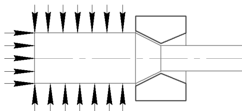
Рис. 2. Обычный способ гидропрессования
